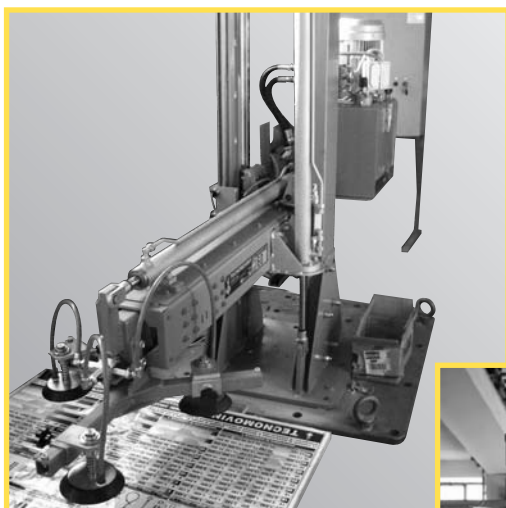
Braccio alimentazione pressa.
